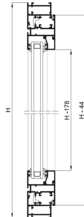
Sección B-B'
